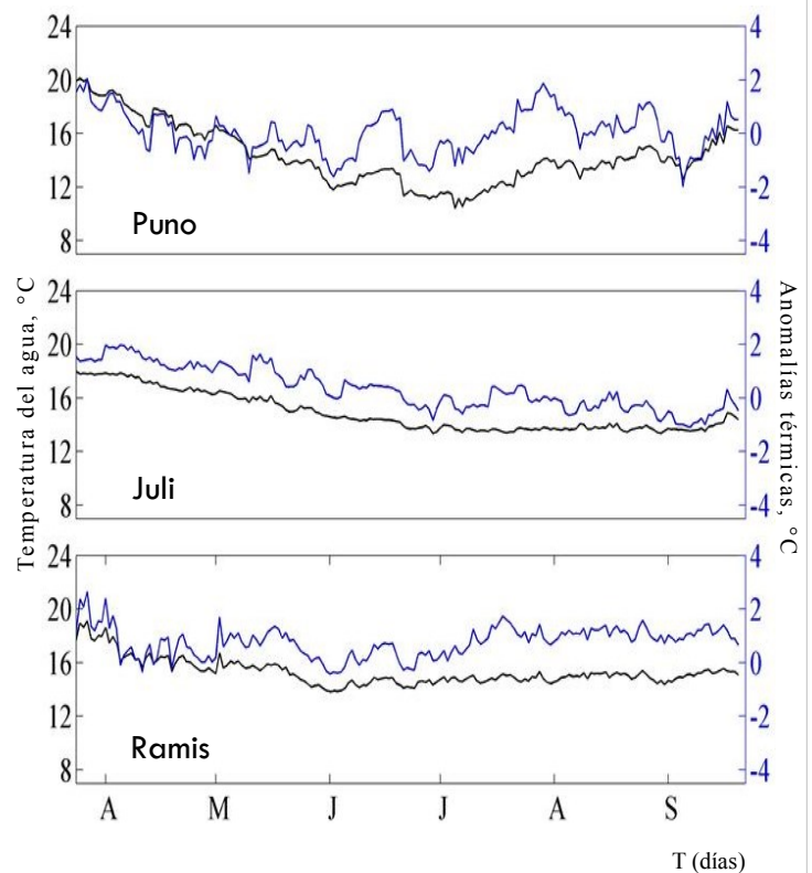
Figura 2. Series de tiempo de la temperatura superficial del agua (°C, línea de color negro) y sus anomalías (°C, línea de color azul) en estaciones del Lago Titicaca para los últimos seis meses al 20 de setiembre de 2016.
