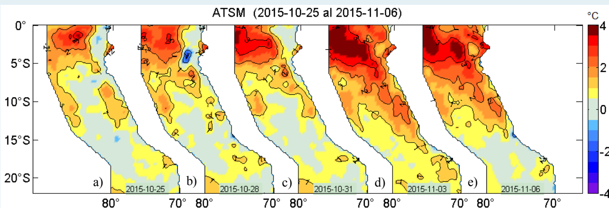
Figura 2. Anomalías de la temperatura superficial del agua (°C) en el mar peruano, cada tres días, entre el 25 de octubre y 06 de noviembre de 2015. Datos: AVHRR/NOAA. Procesamiento: IMARPE.
