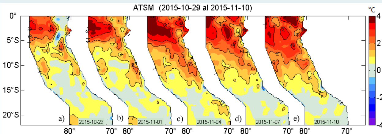
Figura 2. Anomalías de la temperatura superficial del agua (°C) en el mar peruano, cada tres días, entre el 29 de octubre y 10 de noviembre de 2015. Datos: AVHRR/NOAA. Procesamiento: IMARPE.
