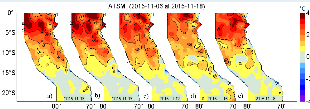
Figura 2. Anomalías de la temperatura superficial del agua (°C) en el mar peruano, cada tres días, entre el 06 al 18 de noviembre de 2015. Datos: AVHRR/NOAA. Procesamiento: IMARPE.
