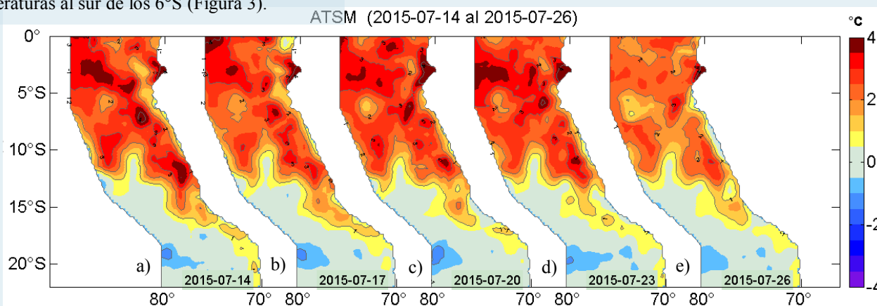
Figura 2. Anomalías de la temperatura superficial del agua ( ^{\circ}\text{C} ) en el mar peruano los días a) 14, b) 17, c) 20, d) 23 y e) 26 de julio. Datos: AVHRR/NOAA. Procesamiento: IMARPE.
