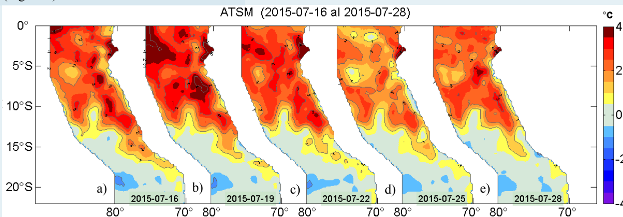
Figura 2. Anomalías de la temperatura superficial del agua (°C) en el mar peruano los días a) 16, b) 19, c) 22, d) 25 y e) 28 de julio. Datos: AVHRR/NOAA. Procesamiento: IMARPE.
