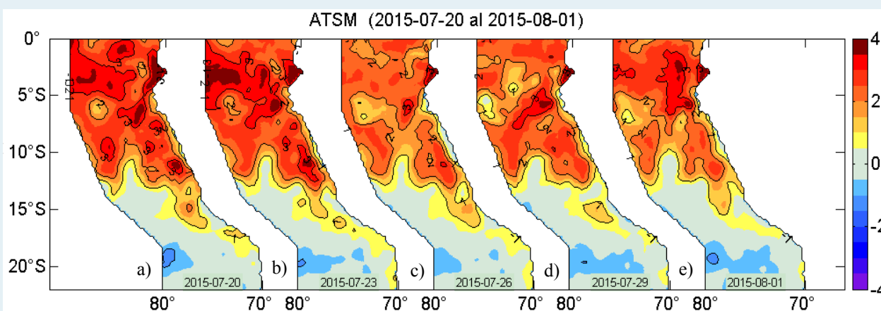
Figura 2. Anomalías de la temperatura superficial del agua (°C) en el mar peruano los días a) 20, b) 23, c) 26, d) 29 de julio y e) 01 de agosto. Datos: AVHRR/NOAA. Procesamiento: IMARPE.
