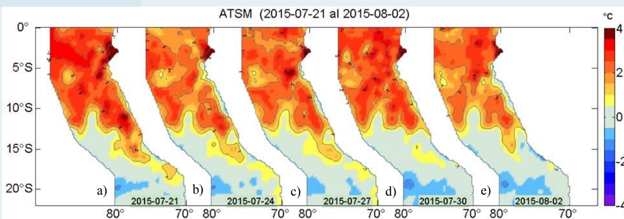
Figura 2. Anomalías de la temperatura superficial del agua (°C) en el mar peruano los días a) 21, b) 24, c) 27, d) 30 de julio y e) 02 de agosto. Datos: AVHRR/NOAA. Procesamiento: IMARPE.
