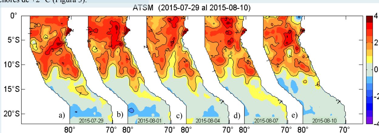
Figura 2. Anomalías de la temperatura superficial del agua (°C) en el mar peruano los días a) 29 de julio, b) 01, c) 04, d) 07, y e) 10 de agosto. Datos: AVHRR/NOAA. Procesamiento: IMARPE.
