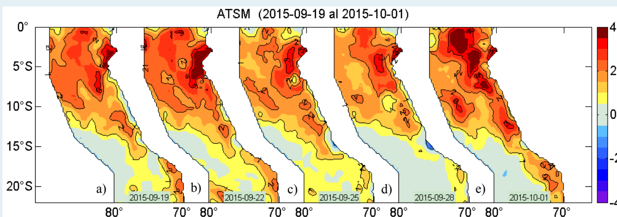
Figura 2. Anomalías de la temperatura superficial del agua (°C) en el mar peruano los días a) 19, b) 22 c) 25, d) 28 de setiembre y e) 01 de octubre. Datos: AVHRR/NOAA. Procesamiento: IMARPE.
