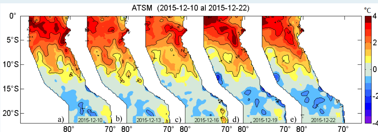
Figura 2. Anomalías de la temperatura superficial del agua (°C) en el mar peruano, cada tres días, entre el 10 y 22 de diciembre de 2015. Datos: AVHRR/NOAA. Procesamiento: IMARPE.
