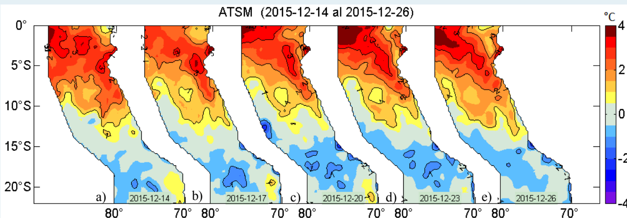
Figura 2. Anomalías de la temperatura superficial del agua (°C) en el mar peruano, cada tres días, entre el 14 y 26 de diciembre de 2015. Datos: AVHRR/NOAA. Procesamiento: IMARPE.
