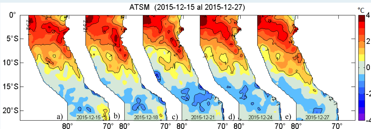
Figura 2. Anomalías de la temperatura superficial del agua (°C) en el mar peruano, cada tres días, entre el 15 y 27 de diciembre de 2015. Datos: AVHRR/NOAA. Procesamiento: IMARPE.
