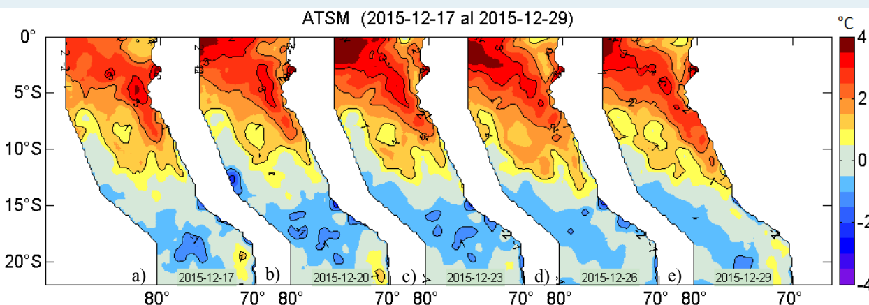
Figura 2. Anomalías de la temperatura superficial del agua (°C) en el mar peruano, cada tres días, entre el 17 y 29 de diciembre de 2015. Datos: AVHRR/NOAA. Procesamiento: IMARPE.
