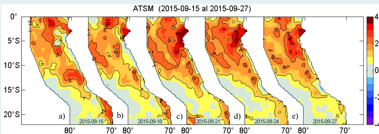
Figura 2. Anomalías de la temperatura superficial del agua ( ^{\circ}\text{C} ) en el mar peruano los días a) 15, b) 18, c) 21, d) 24, y e) 27 de setiembre. Datos: AVHRR/NOAA. Procesamiento: IMARPE.
