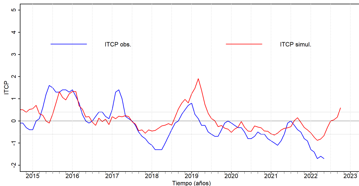
Figura 5. Pronóstico del ITCP mediante un modelo empírico, con datos actualizados hasta el mes de junio del 2022.
