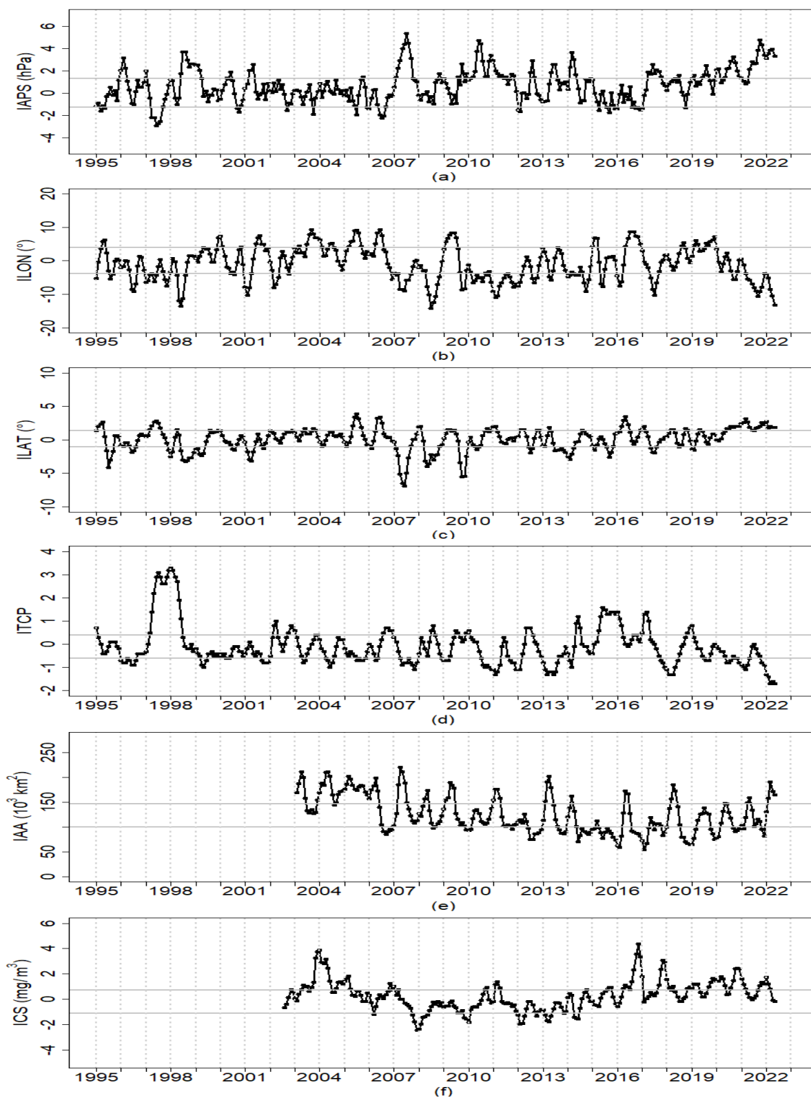
Figura 1. Variación interanual con datos actualizados hasta el mes de junio del 2022 de: (a) Índice del APS (IAPS), (b) Índice de desplazamiento longitudinal del APS (ILON), (c) Índice de desplazamiento
