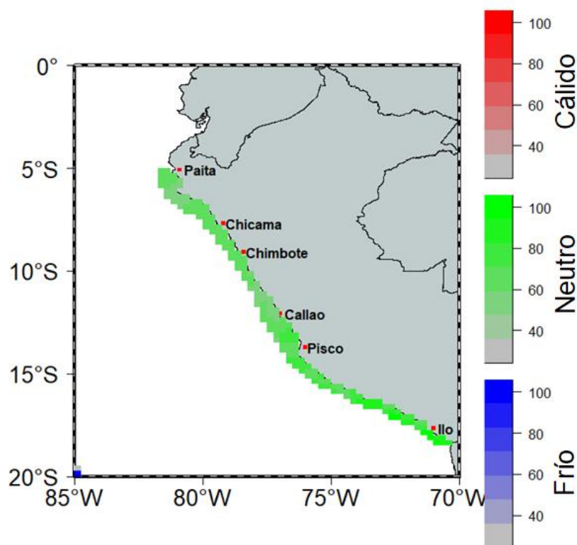
Figura 7. Pronóstico probabilístico espacial para el trimestre JAS 2022 usando un modelo basado en tablas de contingencia.
