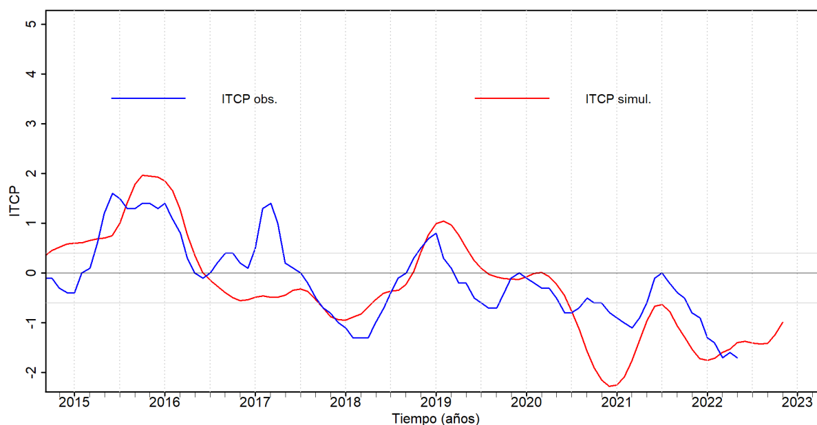
Figura 6. Pronóstico del ITCP mediante el modelo acoplado océano-atmósfera de complejidad intermedia con datos actualizados hasta el mes de junio del 2022.
