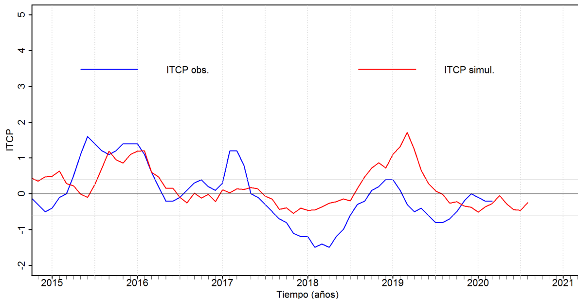
Figura 5. Pronóstico del ITCP mediante un modelo empírico, con datos actualizados hasta el mes de abril del 2020.
