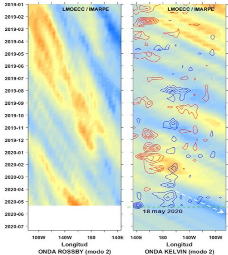
Figura 4. Diagrama Hovmöller longitud-tiempo de Ondas Rossby simuladas ( 3^{\circ} - 5^{\circ} S) y de Ondas Kelvin Ecuatoriales simuladas de modo baroclínico 2 (líneas punteadas), en el Pacífico Ecuatorial ( 0^{\circ} N), anomalías positivas (contornos rojos) y negativas (contornos azules) del esfuerzo del viento zonal. La línea discontinua horizontal indica el inicio del pronóstico. Se presentan las ondas de hundimiento “cálidas” (flechas negras), y las ondas de afloramiento “frías” (flechas blancas).
