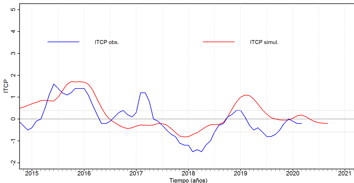
Figura 6. Pronóstico del ITCP mediante el modelo acoplado océano-atmósfera de complejidad intermedia con datos actualizados hasta el mes de abril del 2020.
