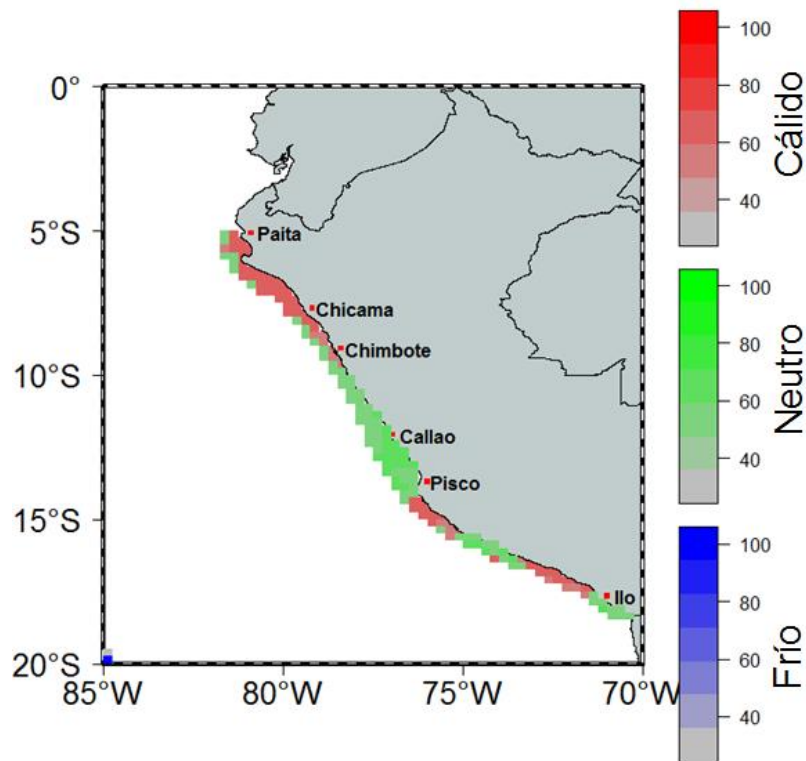
Figura 7. Pronóstico probabilístico espacial para el trimestre MJJ 2020 usando un modelo basado en tablas de contingencia.
