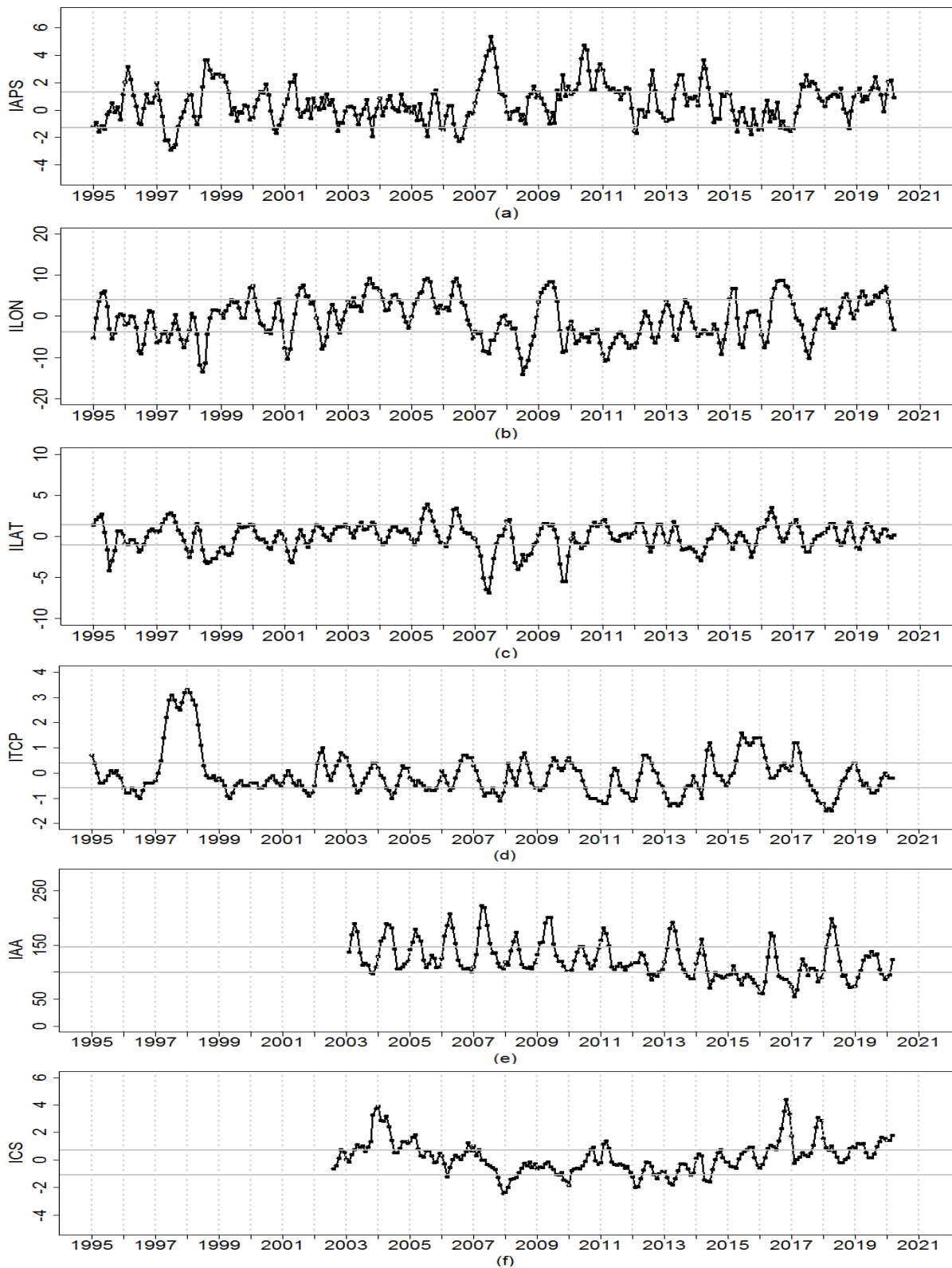
Figura 1. Variación interanual con datos actualizados hasta el mes de abril del 2020 de: (a) Índice del APS (IAPS), (b) Índice de desplazamiento longitudinal del APS (ILON), (c) Índice de desplazamiento latitudinal del APS (ILAT), (d) Índice Térmico Costero Peruano (ITCP), (e) Índice del área de afloramiento (IAA) y (f) Índice de Clorofila a Superficial (ICS).
