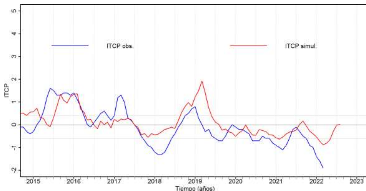
Figura 5. Pronóstico del ITCP mediante un modelo empírico, con datos actualizados hasta el mes de abril del 2022.
