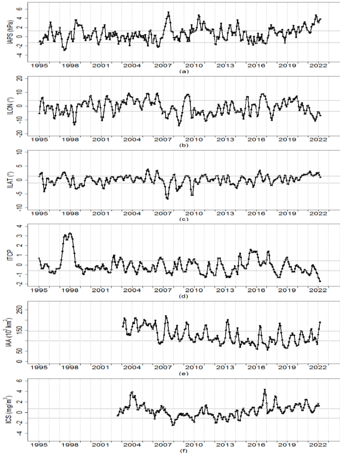
Figura 1. Variación interanual con datos actualizados hasta el mes de abril del 2022 de: (a) Índice del APS (IAPS), (b) Índice de desplazamiento longitudinal del APS (ILON), (c) Índice de desplazamiento latitudinal del APS (ILAT), (d) Índice Térmico Costero Peruano (ITCP), (e) Índice del área de afloramiento (IAA) y (f) Índice de Clorofila a Superficial (ICS).
