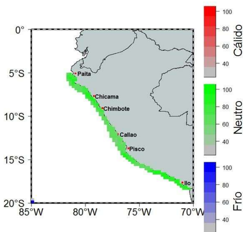
Figura 7. Pronóstico probabilístico espacial para el trimestre MJJ 2022 usando un modelo basado en tablas de contingencia.
