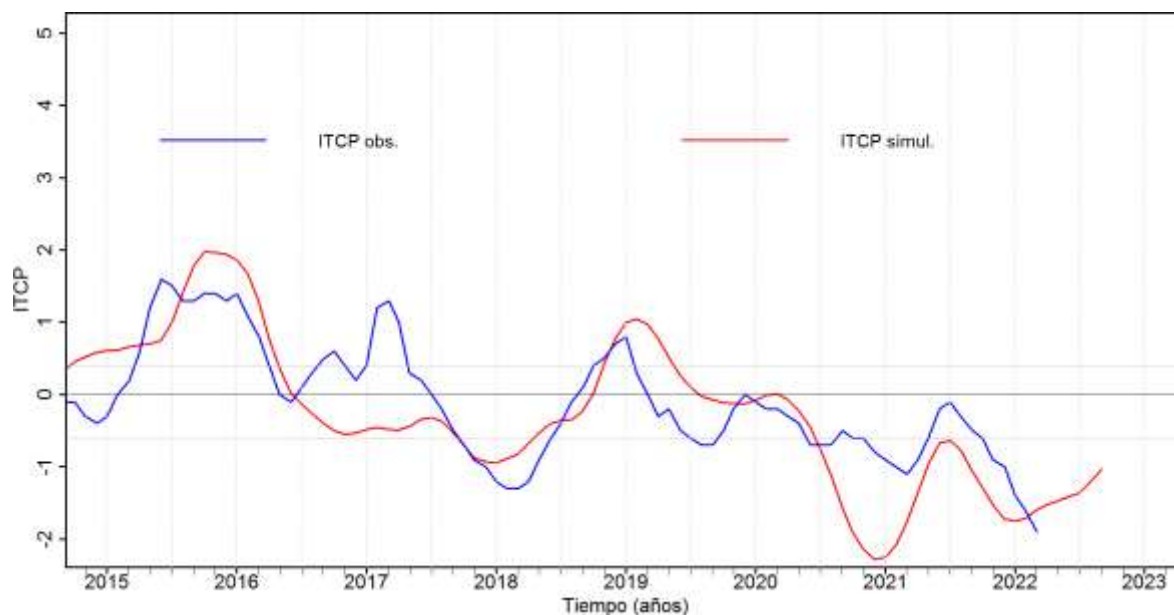
Figura 6. Pronóstico del ITCP mediante el modelo acoplado océano-atmósfera de complejidad intermedia con datos actualizados hasta el mes de abril del 2022.
