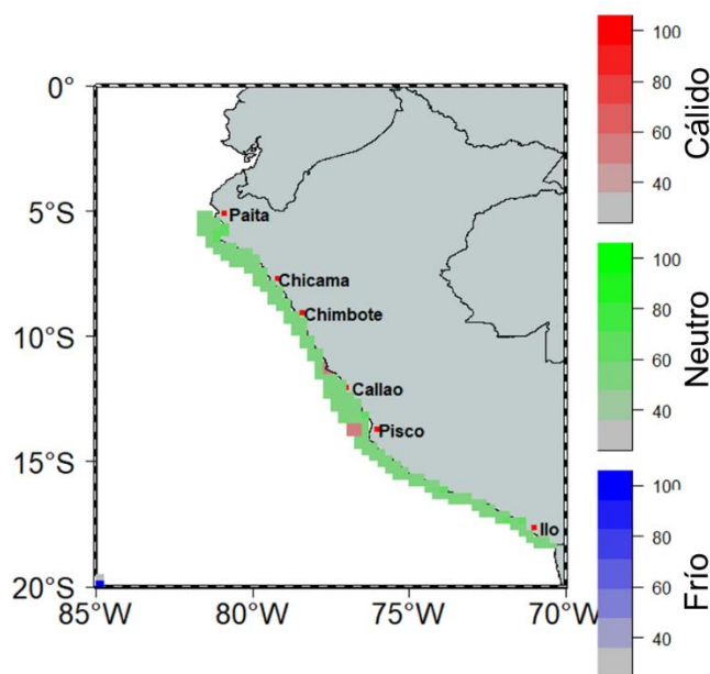
Figura 7. Pronóstico probabilístico espacial para el trimestre EFM 2024 usando un modelo basado en tablas de contingencia.
