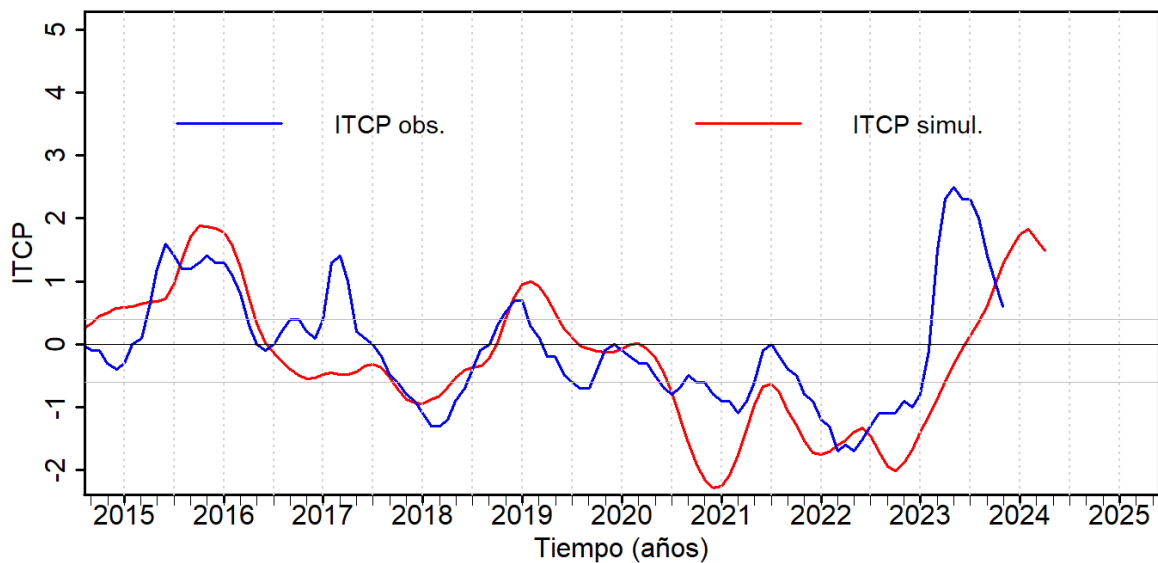
Figura 6. Pronóstico del ITCP mediante el modelo acoplado océano-atmósfera de complejidad intermedia con datos actualizados hasta el mes de diciembre del 2023.
