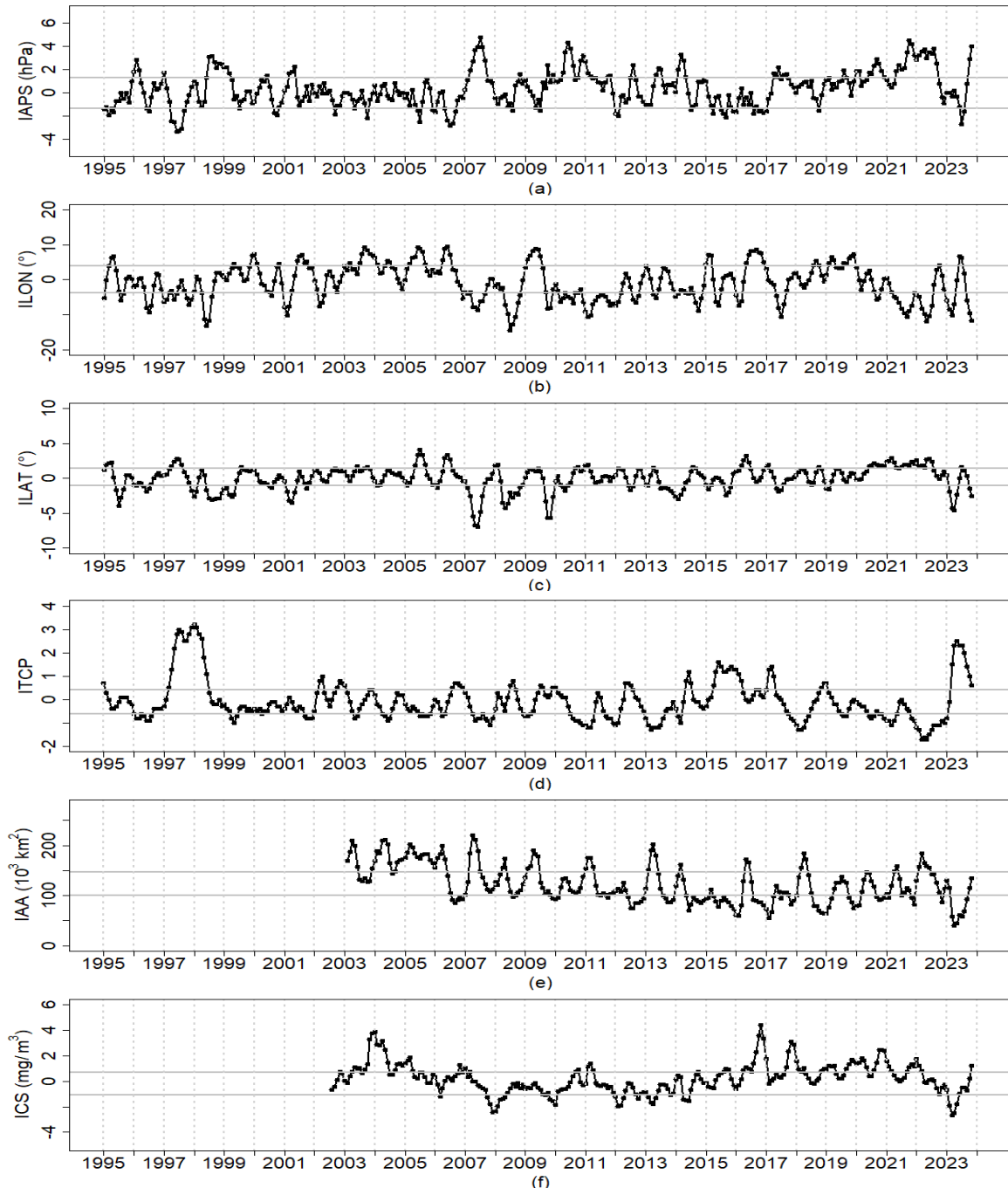
Figura 1. Variación interanual con datos actualizados hasta el mes de diciembre del 2023 de: (a) Índice del APS (IAPS), (b) Índice de desplazamiento longitudinal del APS (ILON), (c) Índice de desplazamiento latitudinal del APS (ILAT), (d) Índice Térmico Costero Peruano (ITCP), (e) Índice del área de afloramiento (IAA) y (f) Índice de Clorofila a Superficial (ICS).
