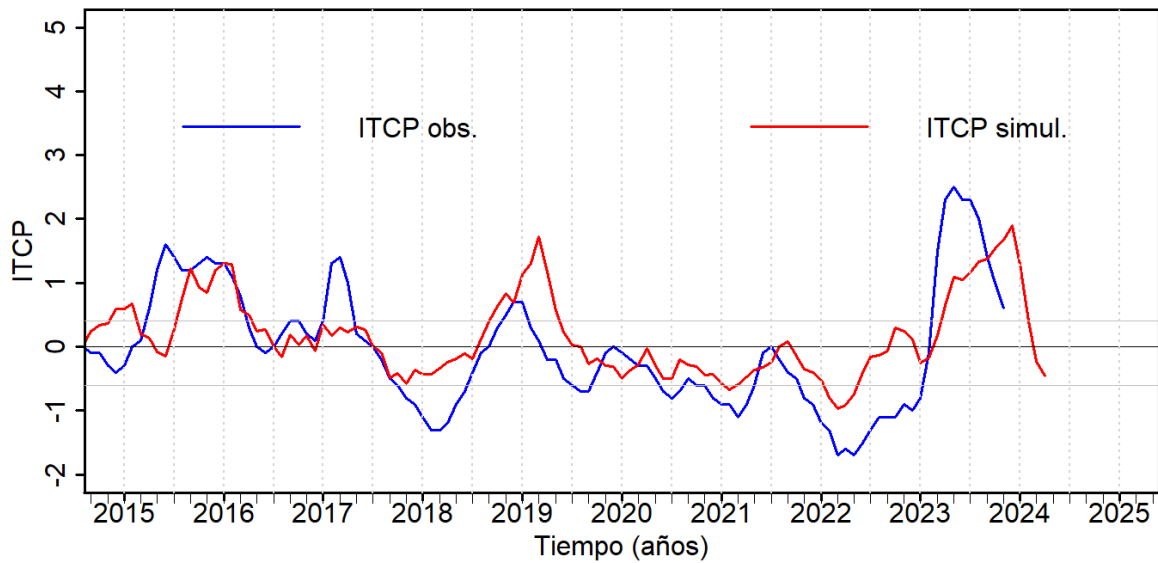
Figura 5. Pronóstico del ITCP mediante un modelo empírico, con datos actualizados hasta el mes de diciembre del 2023.
