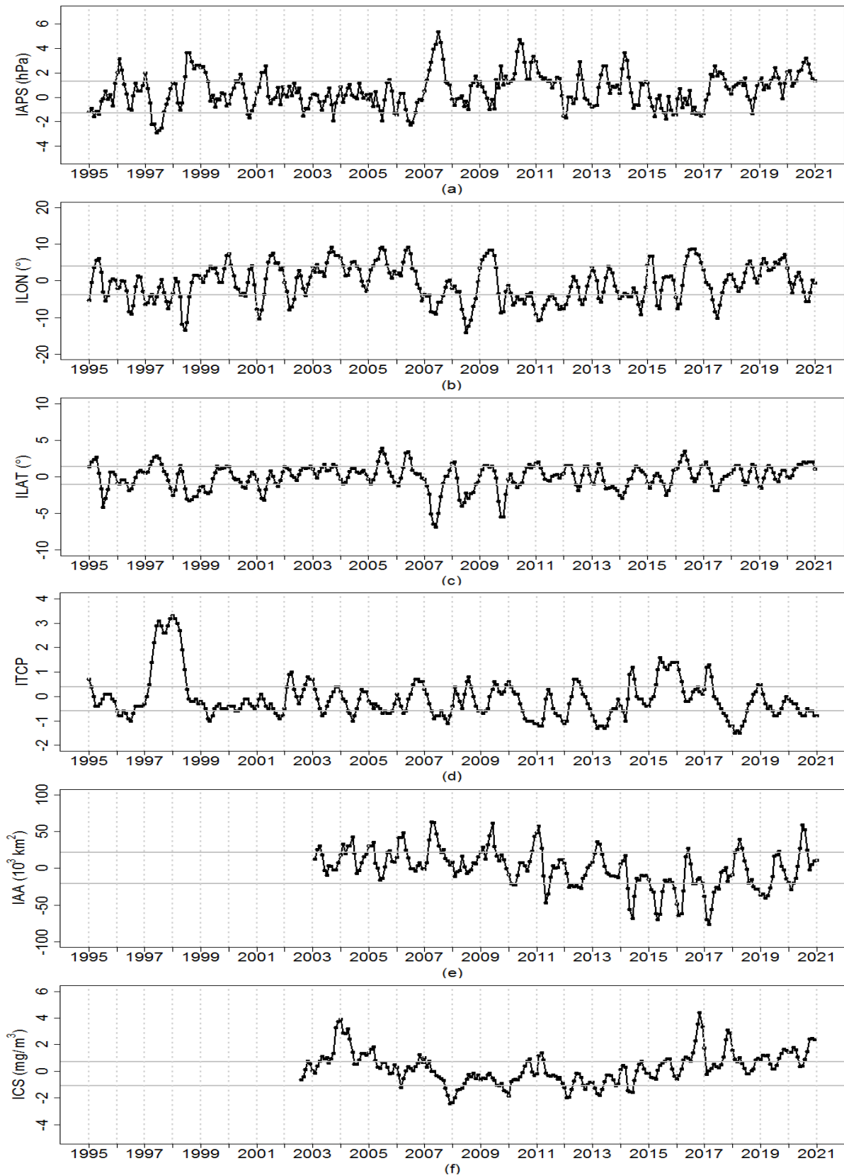
Figura 1. Variación interanual con datos actualizados hasta el mes de febrero del 2021 de: (a) Índice del APS (IAPS), (b) Índice de desplazamiento longitudinal del APS (ILON), (c) Índice de desplazamiento latitudinal del APS (ILAT), (d) Índice Térmico Costero Peruano (ITCP), (e) Índice del área de afloramiento (IAA) y (f) Índice de Clorofila a Superficial (ICS).
