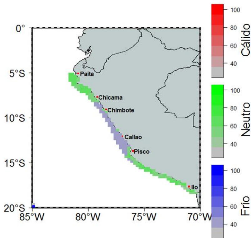
Figura 7. Pronóstico probabilístico espacial para el trimestre MAM 2021 usando un modelo basado en tablas de contingencia.
