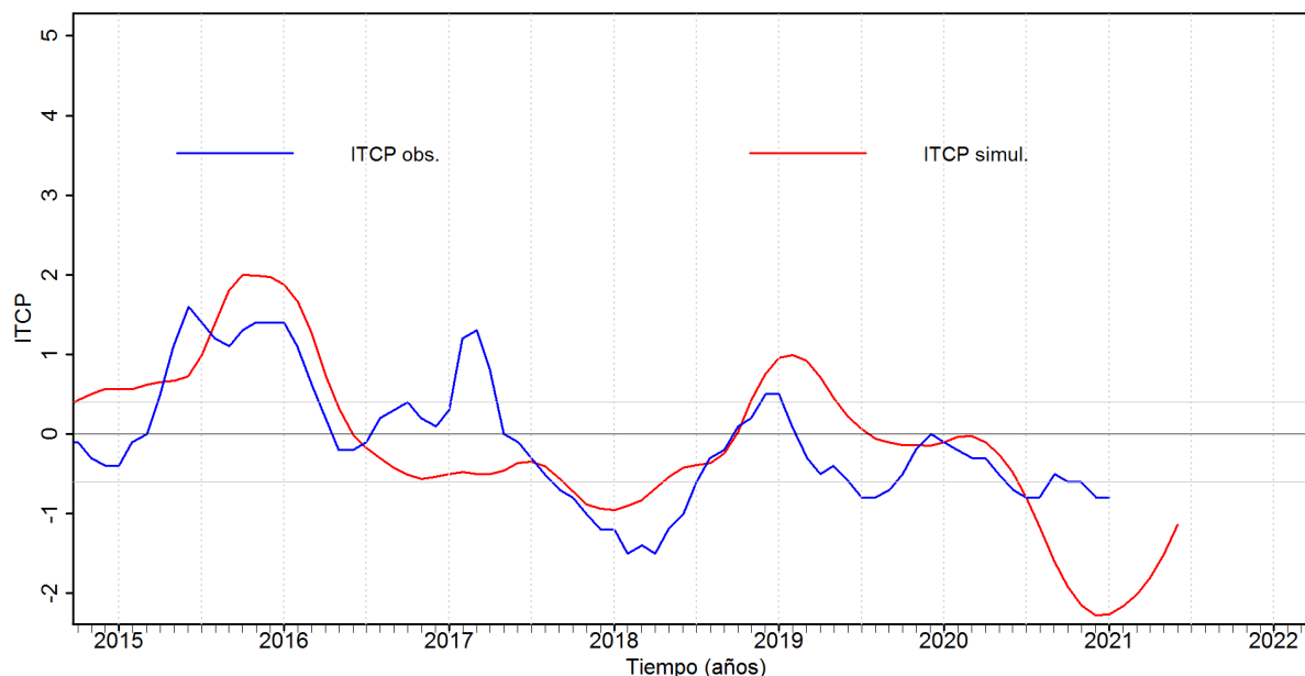
Figura 6. Pronóstico del ITCP mediante el modelo acoplado océano-atmósfera de complejidad intermedia con datos actualizados hasta el mes de febrero del 2021.
