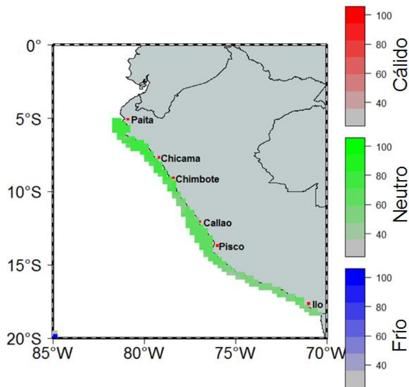
Figura 7. Pronóstico probabilístico espacial para el trimestre ASO 2020 usando un modelo basado en tablas de contingencia.
