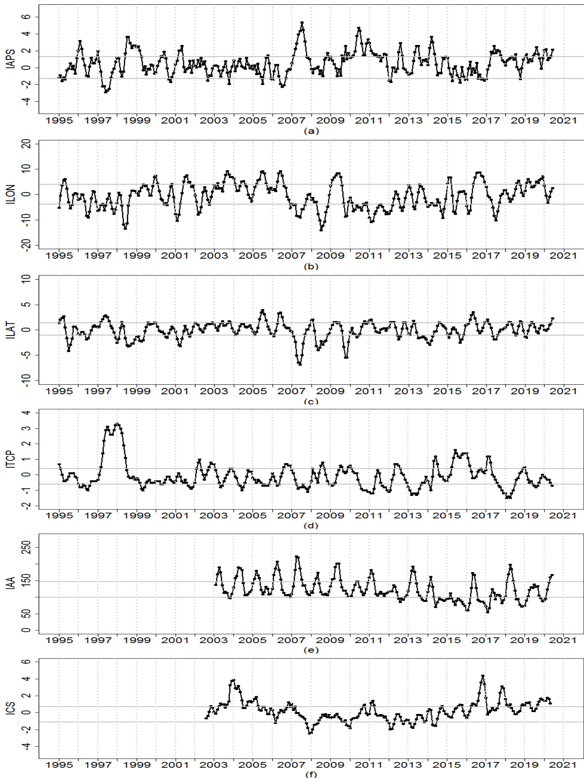
Figura 1. Variación interanual con datos actualizados hasta el mes de julio del 2020 de: (a) Índice del APS (IAPS), (b) Índice de desplazamiento longitudinal del APS (ILON), (c) Índice de desplazamiento latitudinal del APS (ILAT), (d) Índice Térmico Costero Peruano (ITCP), (e) Índice del área de afloramiento (IAA) y (f) Índice de Clorofila a Superficial (ICS).
