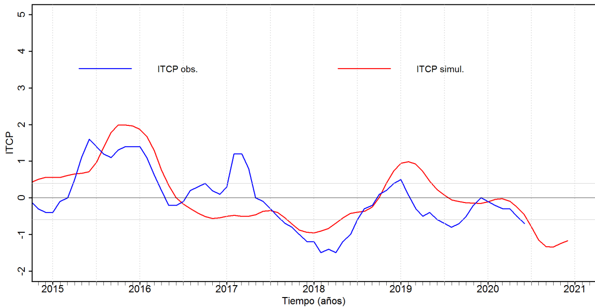
Figura 6. Pronóstico del ITCP mediante el modelo acoplado océano-atmósfera de complejidad intermedia con datos actualizados hasta el mes de julio del 2020.
