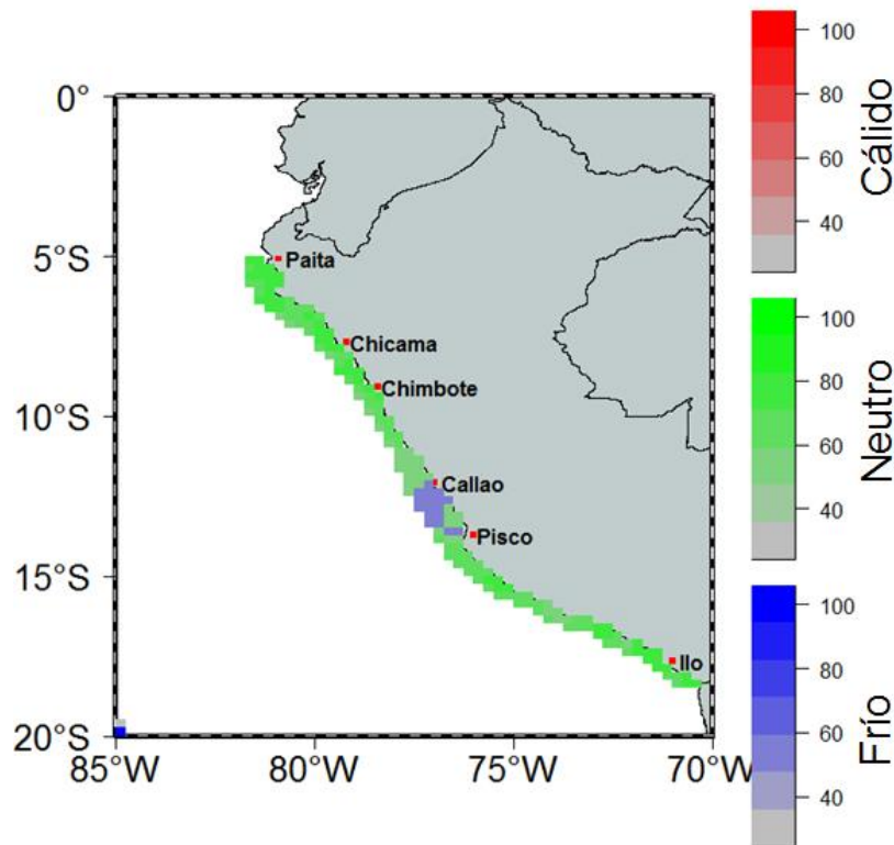
Figura 7. Pronóstico probabilístico espacial para el trimestre AMJ 2022 usando un modelo basado en tablas de contingencia.
