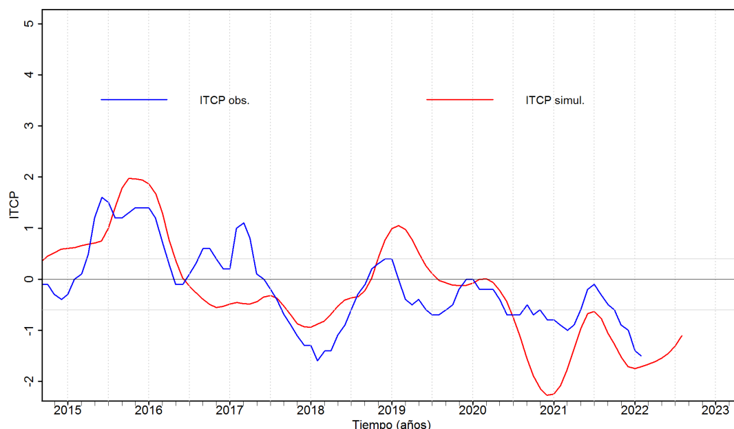
Figura 6. Pronóstico del ITCP mediante el modelo acoplado océano-atmósfera de complejidad intermedia con datos actualizados hasta el mes de marzo del 2022.
