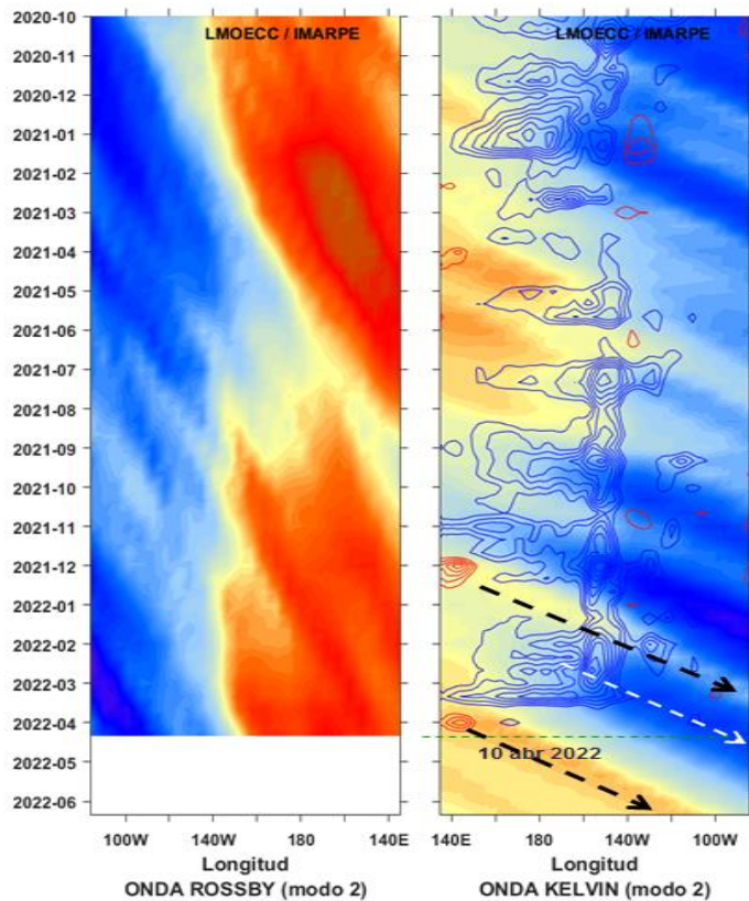
Figura 4. Diagrama Hovmöller longitud-tiempo de Ondas Rossby simuladas (3°-5°S) y de Ondas Kelvin Ecuatoriales simuladas de modo baroclínico 2 (líneas punteadas), en el Pacífico Ecuatorial (0°N), anomalías positivas (contornos rojos) y negativas (contornos azules) del esfuerzo del viento zonal. La línea discontinua horizontal indica el inicio del pronóstico. Se presentan las ondas de hundimiento "cálidas" (flechas negras), y las ondas de afloramiento "frías" (flechas blancas).
