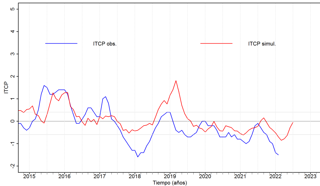
Figura 5. Pronóstico del ITCP mediante un modelo empírico, con datos actualizados hasta el mes de marzo del 2022.
