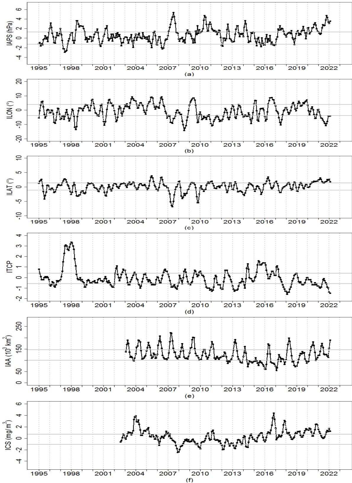
Figura 1. Variación interanual con datos actualizados hasta el mes de marzo del 2022 de: (a) Índice del APS (IAPS), (b) Índice de desplazamiento longitudinal del APS (ILON), (c) Índice de desplazamiento latitudinal del APS (ILAT), (d) Índice Térmico Costero Peruano (ITCP), (e) Índice del área de afloramiento (IAA) y (f) Índice de Clorofila a Superficial (ICS).
