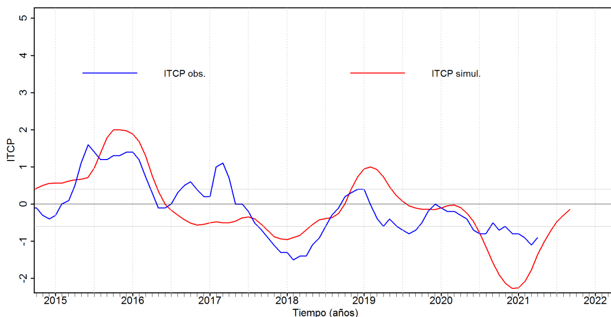
Figura 6. Pronóstico del ITCP mediante el modelo acoplado océano-atmósfera de complejidad intermedia con datos actualizados hasta el mes de mayo del 2021.
