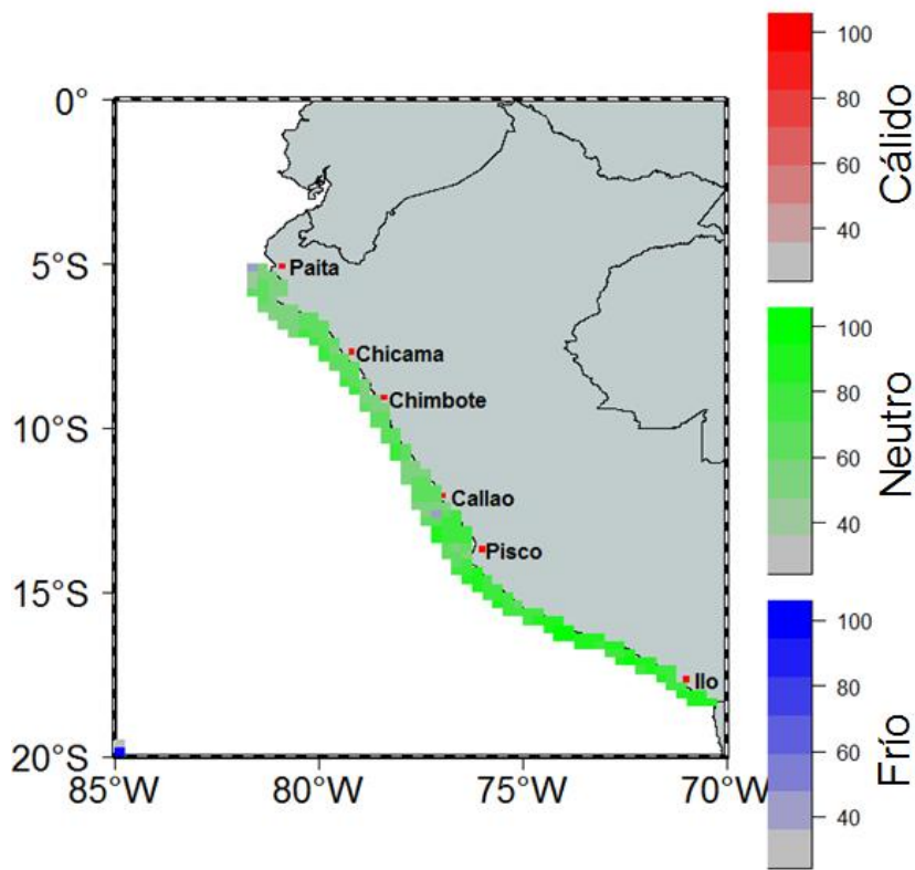
Figura 7. Pronóstico probabilístico espacial para el trimestre JJA 2021 usando un modelo basado en tablas de contingencia.
