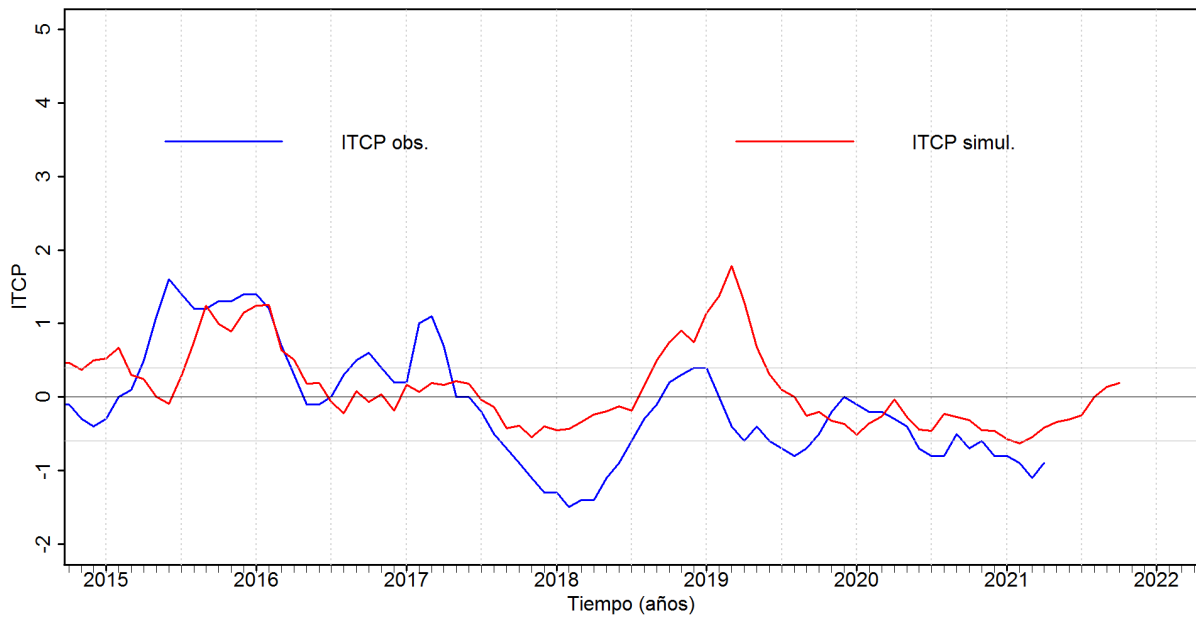
Figura 5. Pronóstico del ITCP mediante un modelo empírico, con datos actualizados hasta el mes de mayo del 2021.
