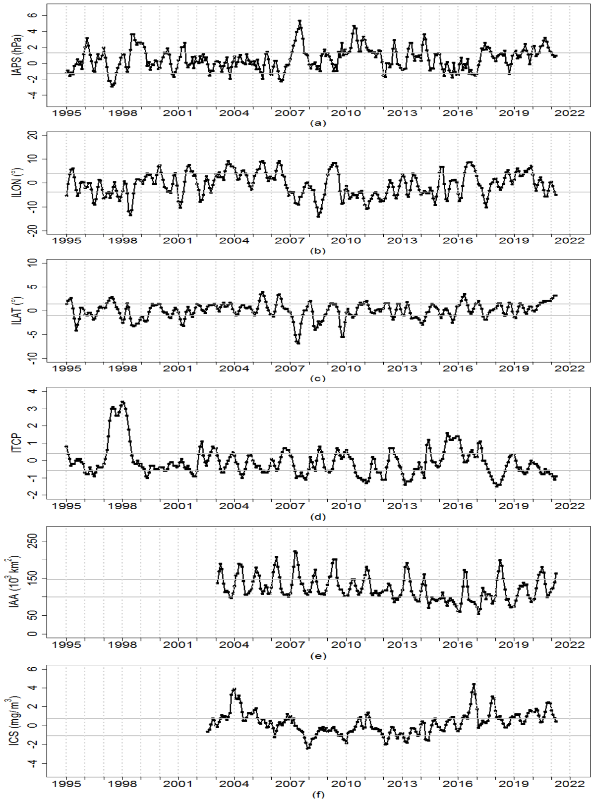
Figura 1. Variación interanual con datos actualizados hasta el mes de mayo del 2021 de: (a) Índice del APS (IAPS), (b) Índice de desplazamiento longitudinal del APS (ILON), (c) Índice de desplazamiento latitudinal del APS (ILAT), (d) Índice Térmico Costero Peruano (ITCP), (e) Índice del área de afloramiento (IAA) y (f) Índice de Clorofila a Superficial (ICS).
