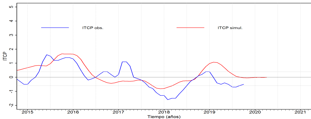
Figura 6. Pronóstico del ITCP mediante el modelo acoplado océano-atmósfera de complejidad intermedia con datos actualizados hasta el mes de noviembre del 2019.
