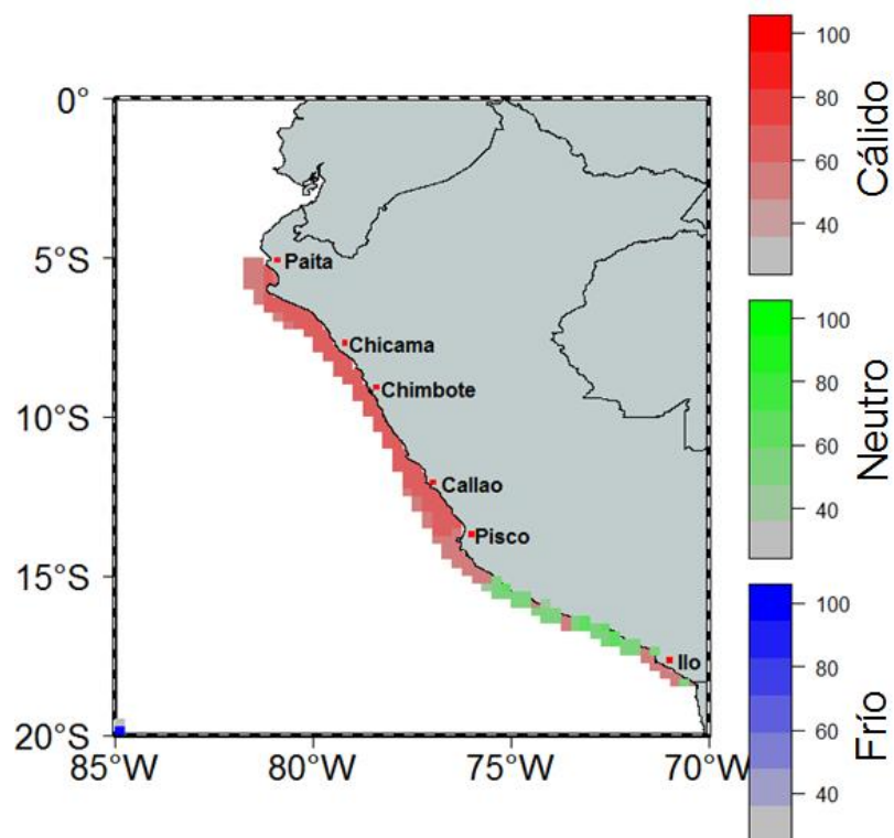
Figura 7. Pronóstico probabilístico espacial para el trimestre DEF 2019-20 usando un modelo basado en tablas de contingencia.
