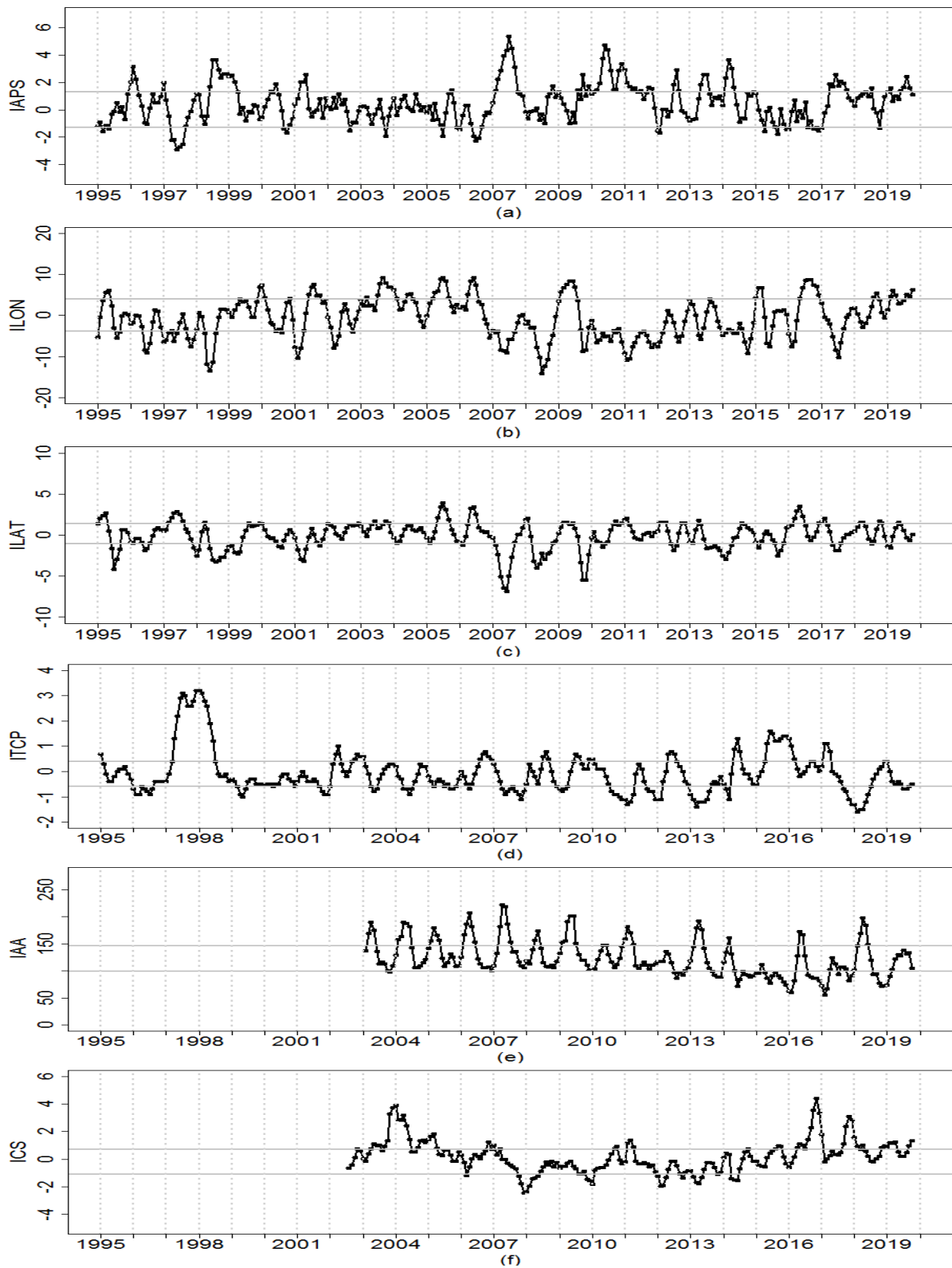
Figura 1. Variación interanual con datos actualizados hasta el mes de noviembre del 2019 de: (a) Índice del APS (IAPS), (b) Índice de desplazamiento longitudinal del APS (ILON), (c) Índice de desplazamiento latitudinal del APS (ILAT), (d) Índice Térmico Costero Peruano (ITCP), (e) Índice del área de afloramiento (IAA) y (f) Índice de Clorofila a Superficial (ICS).
