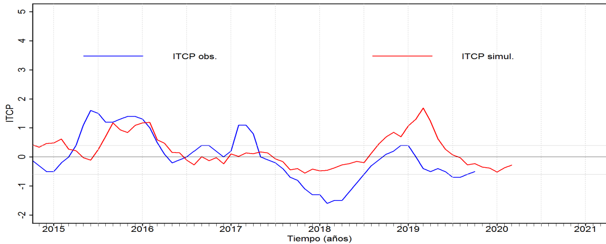
Figura 5. Pronóstico del ITCP mediante un modelo empírico, con datos actualizados hasta el mes de noviembre del 2019.
