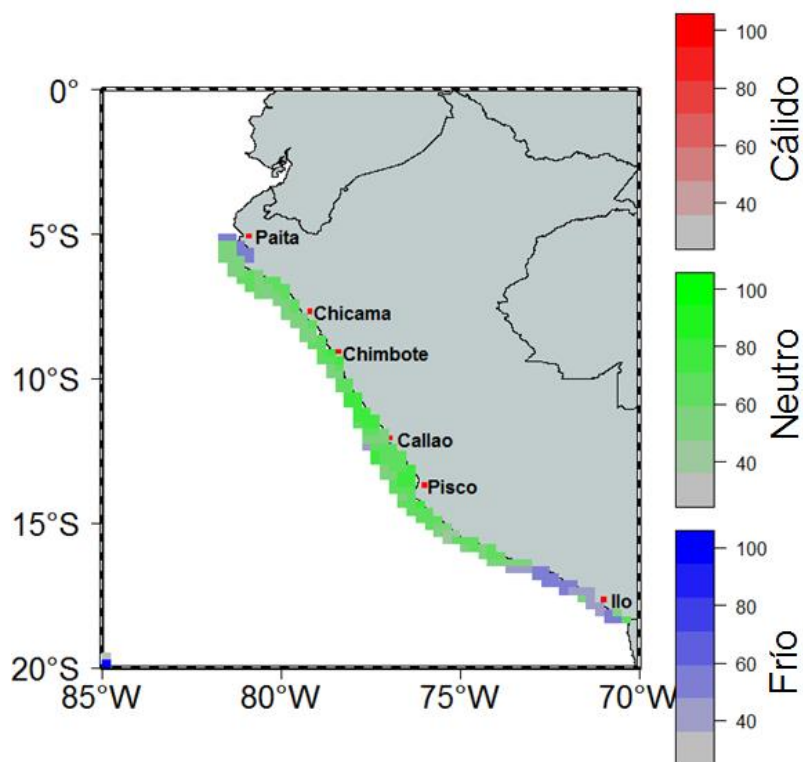
Figura 7. Pronóstico probabilístico espacial para el trimestre NDE 2020-21 usando un modelo basado en tablas de contingencia.
