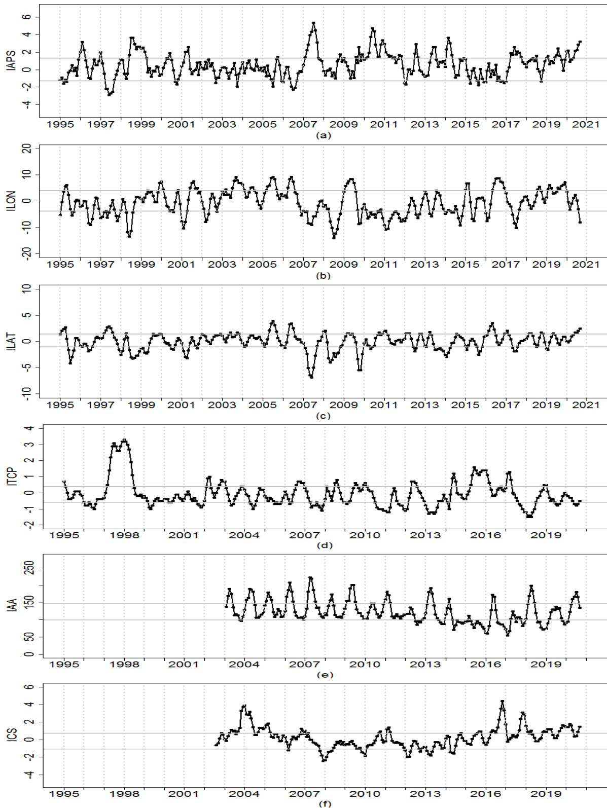
Figura 1. Variación interanual con datos actualizados hasta el mes de octubre del 2020 de: (a) Índice del APS (IAPS), (b) Índice de desplazamiento longitudinal del APS (ILON), (c) Índice de desplazamiento latitudinal del APS (ILAT), (d) Índice Térmico Costero Peruano (ITCP), (e) Índice del área de afloramiento (IAA) y (f) Índice de Clorofila a Superficial (ICS).
