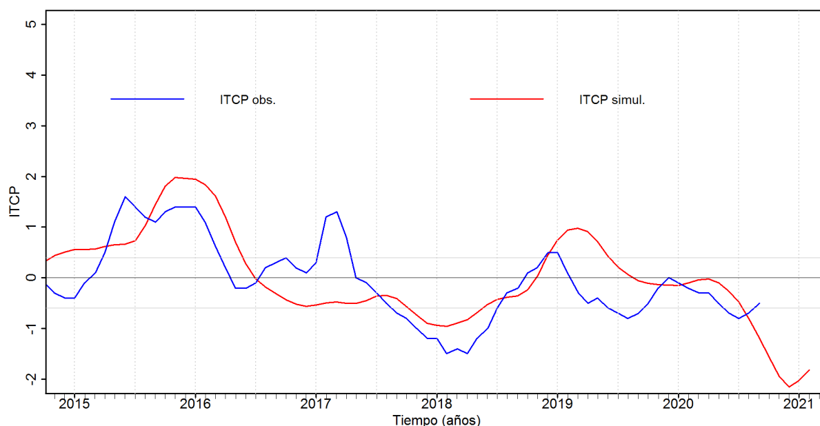
Figura 6. Pronóstico del ITCP mediante el modelo acoplado océano-atmósfera de complejidad intermedia con datos actualizados hasta el mes de octubre del 2020.
