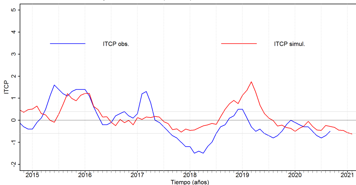
Figura 5. Pronóstico del ITCP mediante un modelo empírico, con datos actualizados hasta el mes de octubre del 2020.
